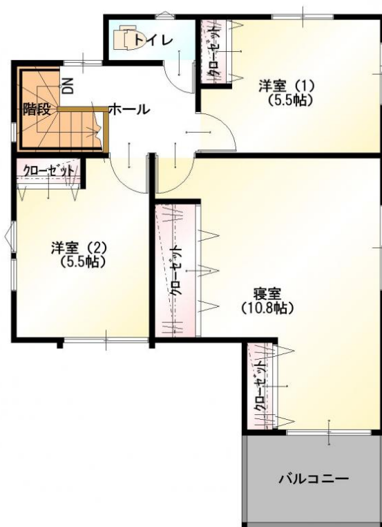
2階
